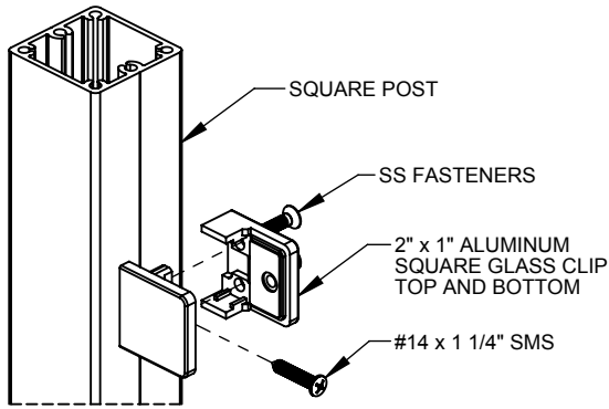
○ OPTION-1 SCALE 1 : 4
