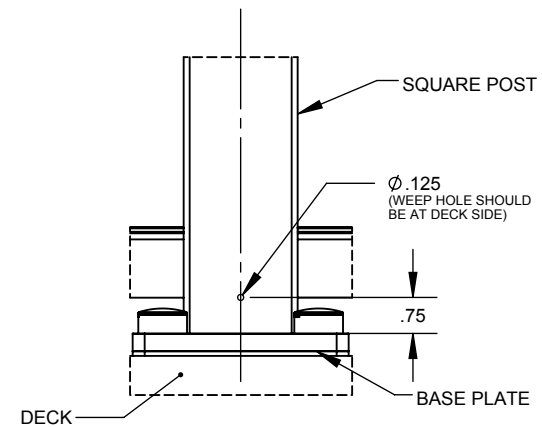
8 TYP. WEEP HOLE
